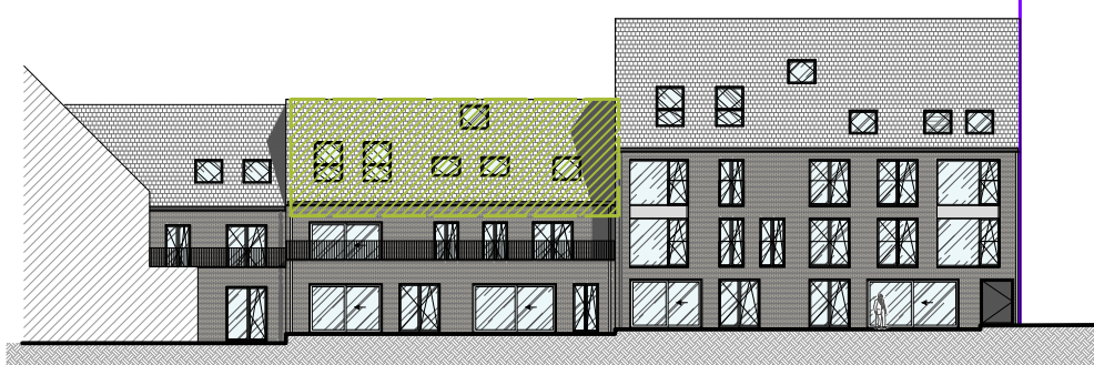
Achtergevel Limbosweg
