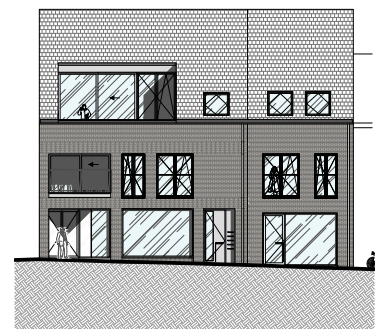
Voorgevel Oudstrijdersplein
