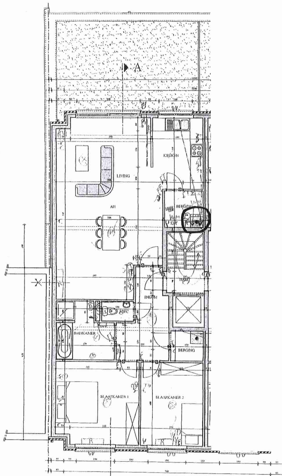
A VERDIEPING 1
