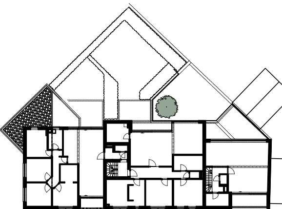
NIVEAU +01
